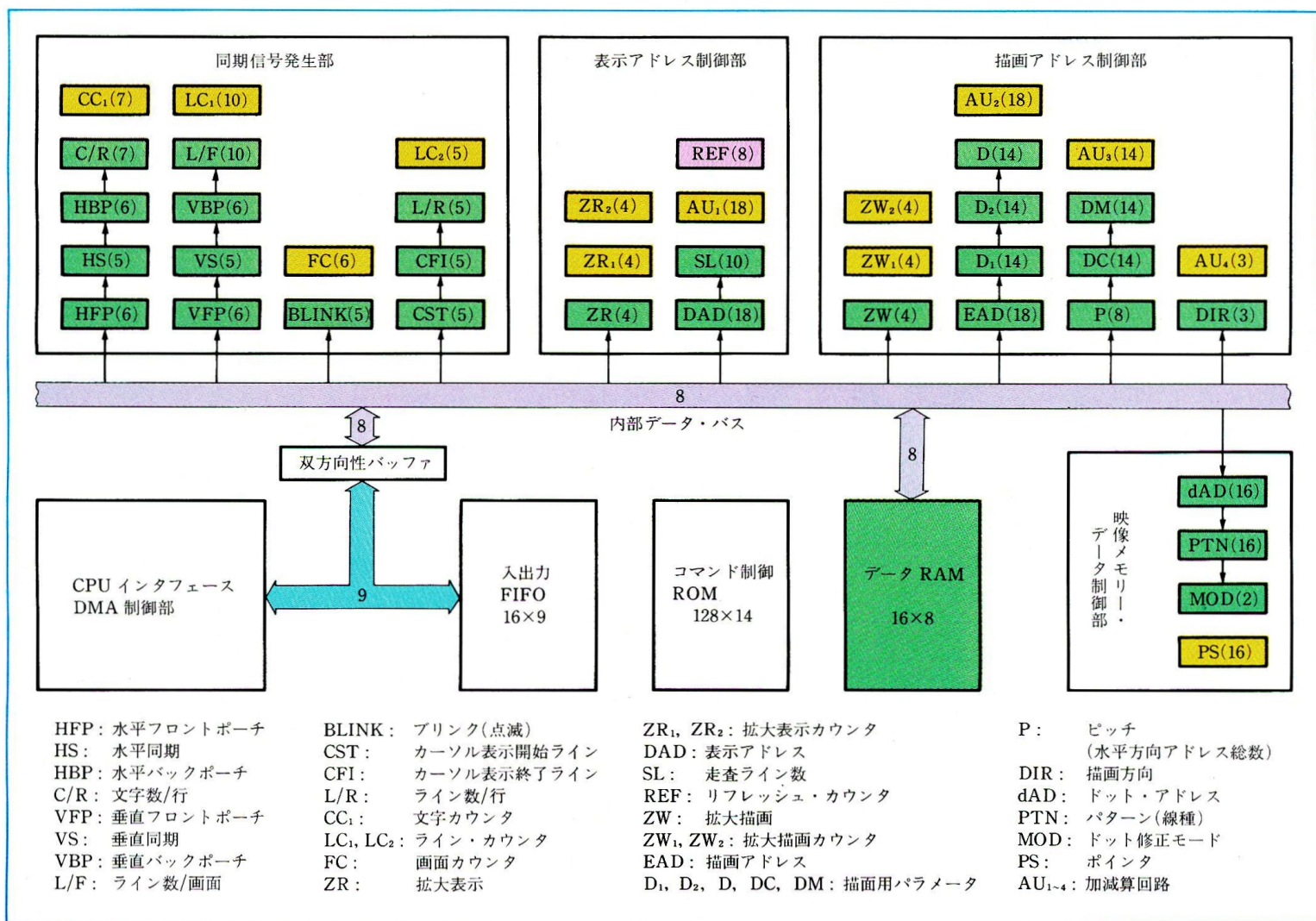
図 2(b) GDC のレジスタ・レベル・ブロック図。従来型 CRTC は同期信号発生部と表示アドレス制御部の一部しか集積していない。■部レジスタはプログラムで任意値に設定できる。各レジスタ群は ■ で示す専用のカウンタや演算器を持ち, 内部データ・バスとは別経路で並列動作する
