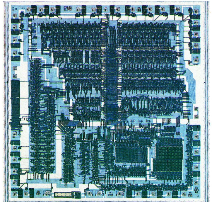
図2(a) GDCチップ。ゲート長 3\mu\text{m} のnチャンネル・シリコン・ゲートE/D MOSトランジスタ1万3000個を搭載する。チップ・サイズは 5.29\times 5.39\text{mm} 。高速並列演算を実行するためハード・ワイアド論理を用いる。規則性のある繰り返し回路にまとも、マスク・レイアウトを容易にしている
