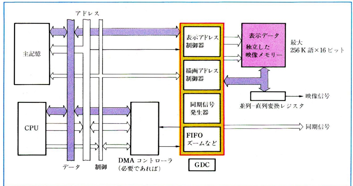
図1 GDCのシステム・ブロック図。GDCおよび映像メモリーはブラック・ボックス化され、独立して動作するI/O機器としてとらえることができ、拡張性に富む
