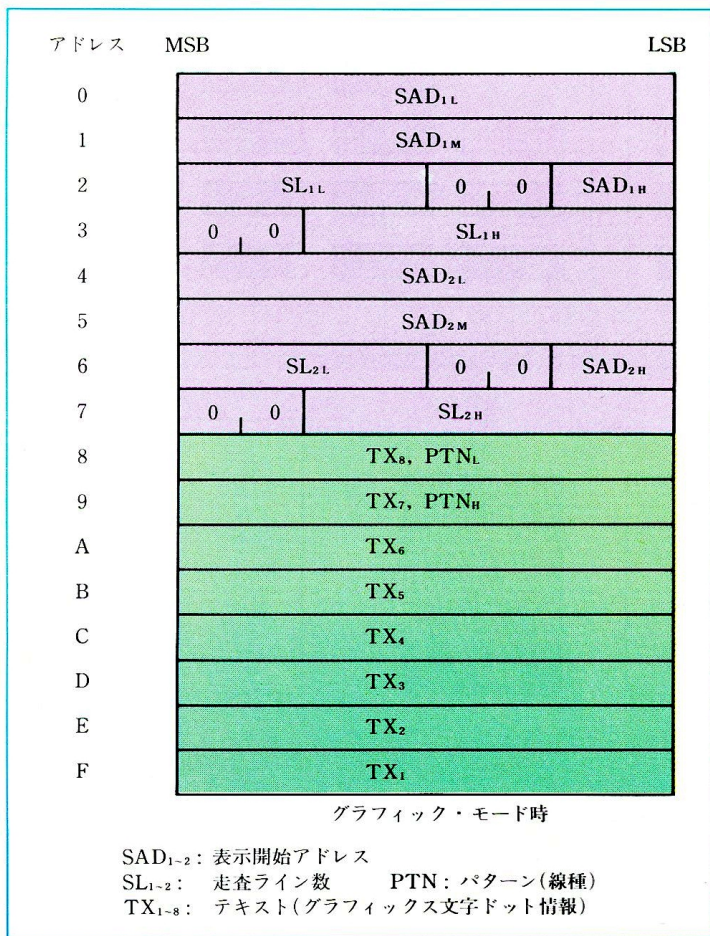
図 3 内蔵データ RAM マップ。コマンドによって任意なアドレスからデータを設定できる。下位 8 バイトは表示用、上位 8 バイトは描画時、線種情報記憶用または文字ドット情報記憶用として使用する
