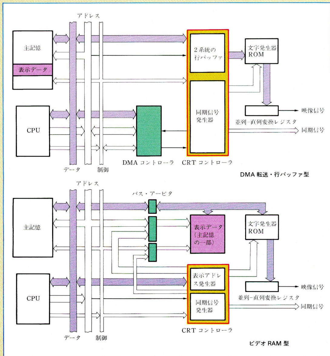
図 A 従来の CRT 制御用 LSI のシステム・ブロック図。両方式共に、表示データは主記憶中にマップされる。システム構成上の自由度や拡張性に乏しい。本文で紹介する GDC の場合は 色部回路が不要となる
